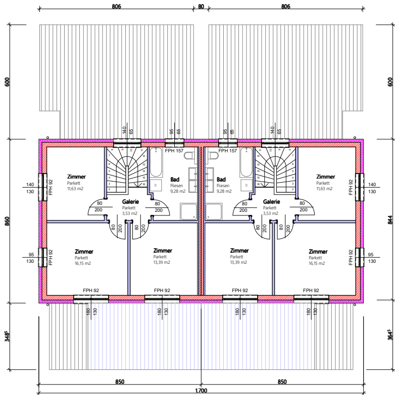
OBERGESCHOSS WNF: 53,98 m 2
