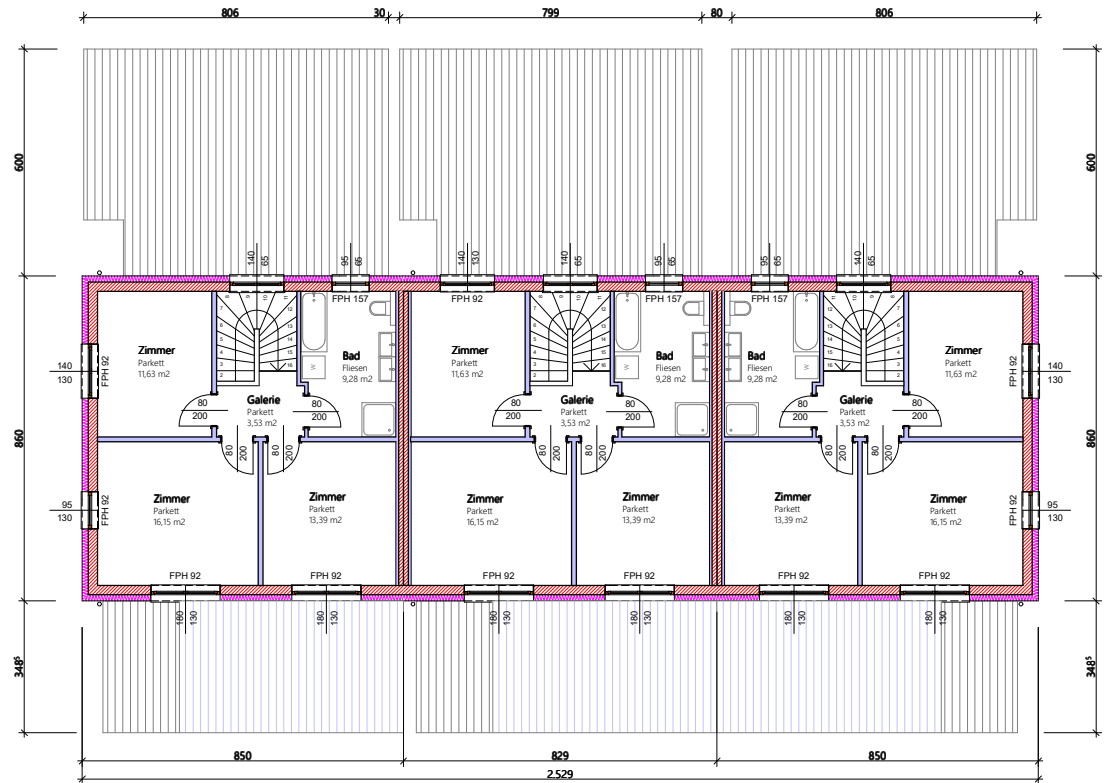
OBERGESCHOSS WNF: 53,98 m 2
